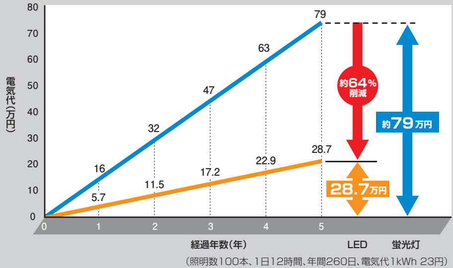
■従来丸形蛍光灯20W+安定器と20W形LEDとの比較
